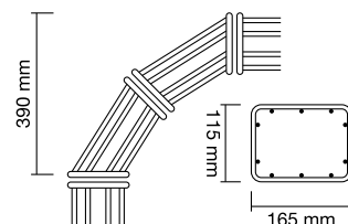
Eckelement 90° – Rechteck 115 / 165 mm
